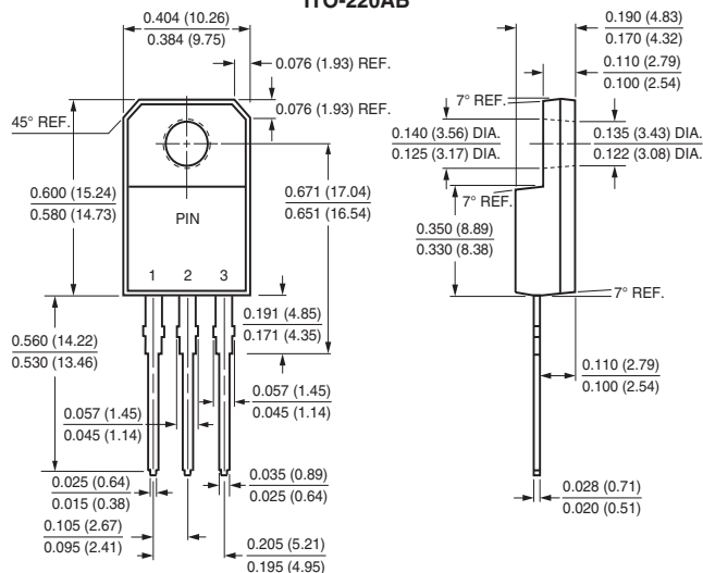
ITO-220AB
