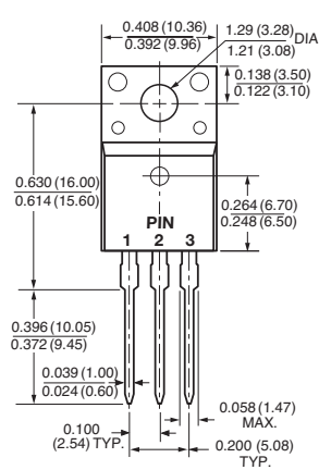
ITO-220AB
