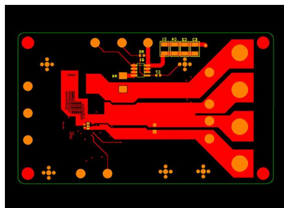
Figure 17. Bottom Layer
