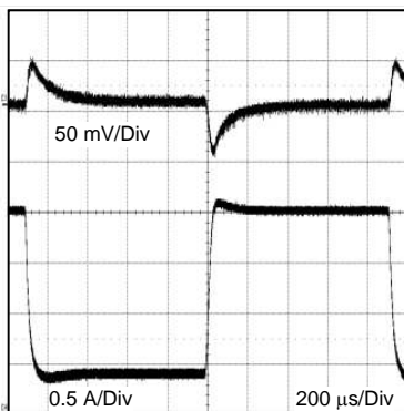
12 V_{IN} 3.3 V_O 0.6-A to 2-A Step
